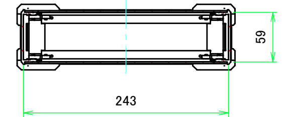
C-C ( 1:4.5 )
