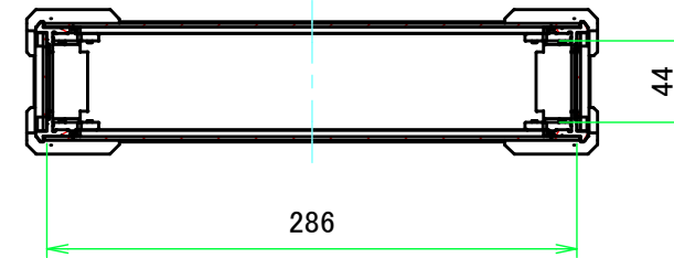
A-A ( 1:4.5 )
