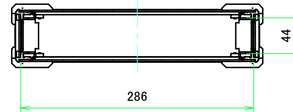
A-A ( 1:4.5 )
