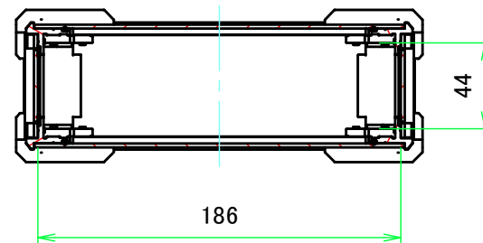
A-A ( 1:3.5 )
