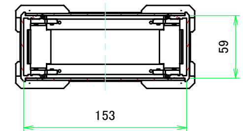
C-C ( 1:3.5 )
