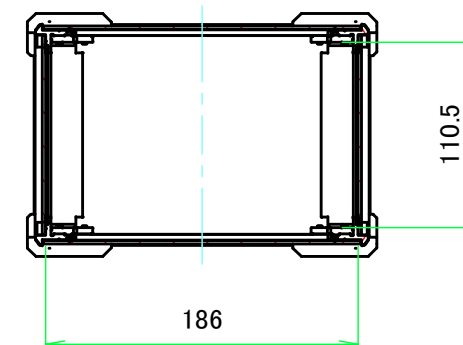
A-A ( 1:4.5 )
