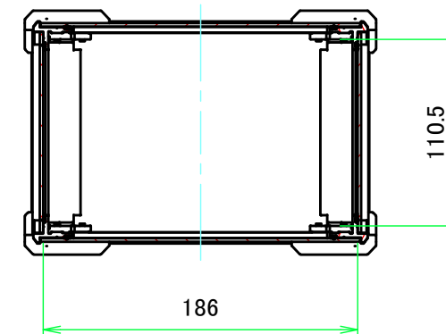
A-A ( 1:4 )
