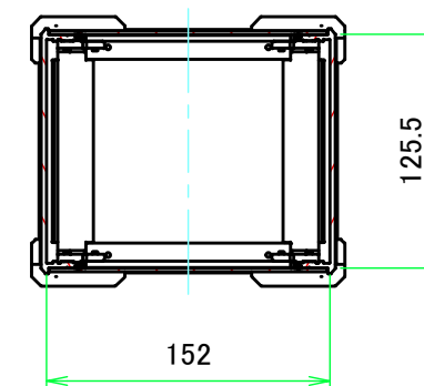
C-C ( 1:4.5 )
