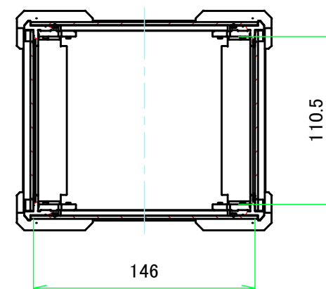
A-A ( 1:3.5 )
