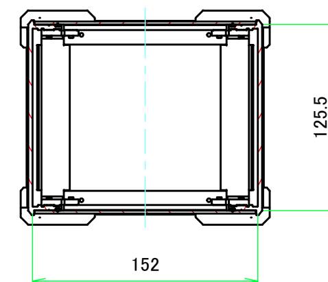
C-C ( 1:3.5 )
