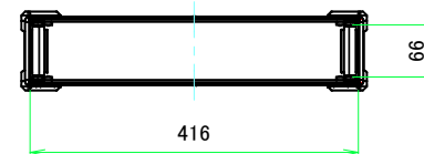
A-A (1:7.5)
