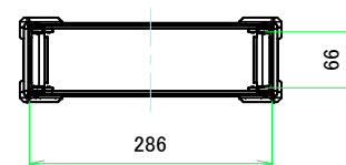
A-A (1:7)
