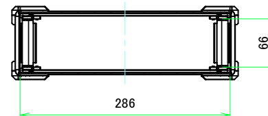
A-A (1:5)
