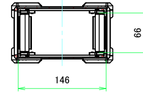
A-A (1:4.5)
