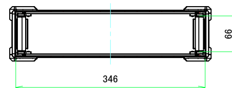
A-A (1:5)
