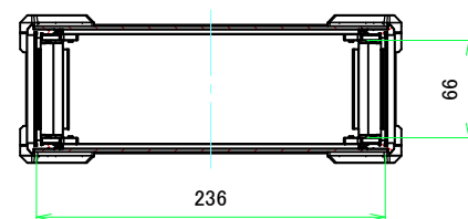
A-A (1:4)
