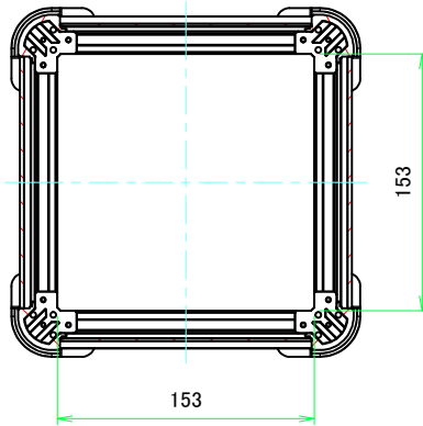
B-B (1:3.5)
