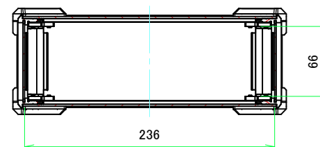
A-A (1:3.5)
