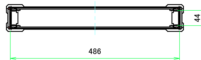
A-A ( 1:6.5 )
