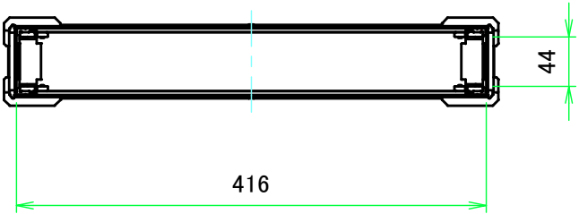
A-A (1:6)
