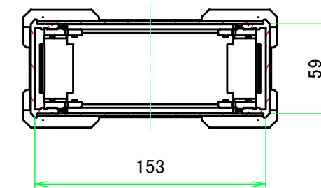
C-C ( 1:3.5 )
