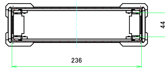
A-A ( 1:3.5 )
