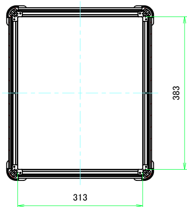
B-B ( 1:6.5 )
