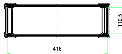
A-A ( 1:6.5 )
