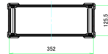
C-C ( 1:6.5 )
