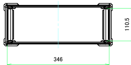
A-A ( 1:5.5 )
