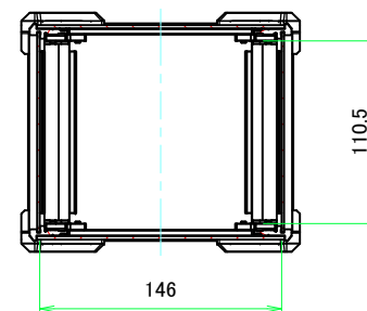
A-A (1:3.5)
