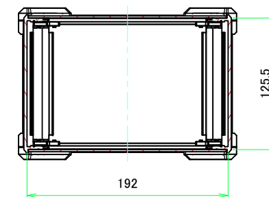
C-C (1:3.5)
