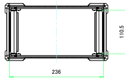
A-A ( 1:4 )
