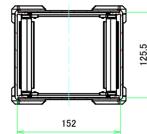
C-C ( 1:4 )
