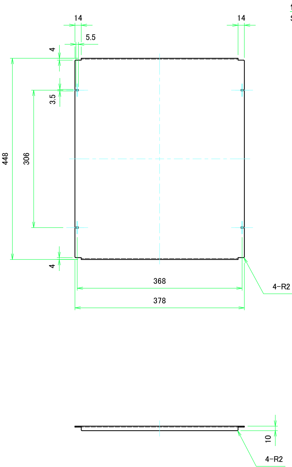
シャーシ / Mounting plate
