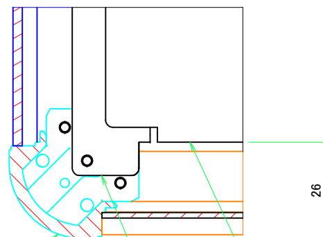
L金具 L-bracket
