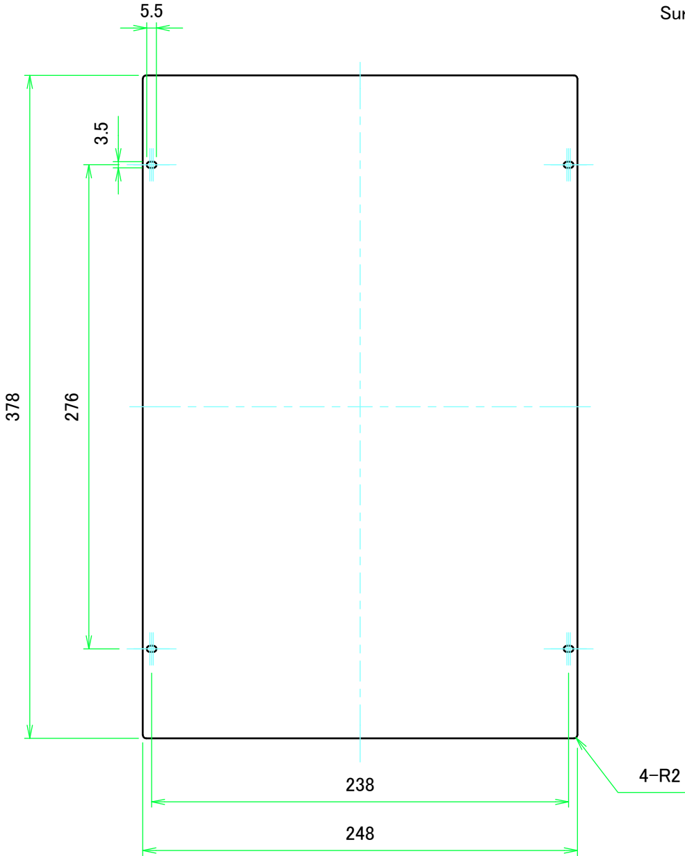
シャーシ / Mounting plate
