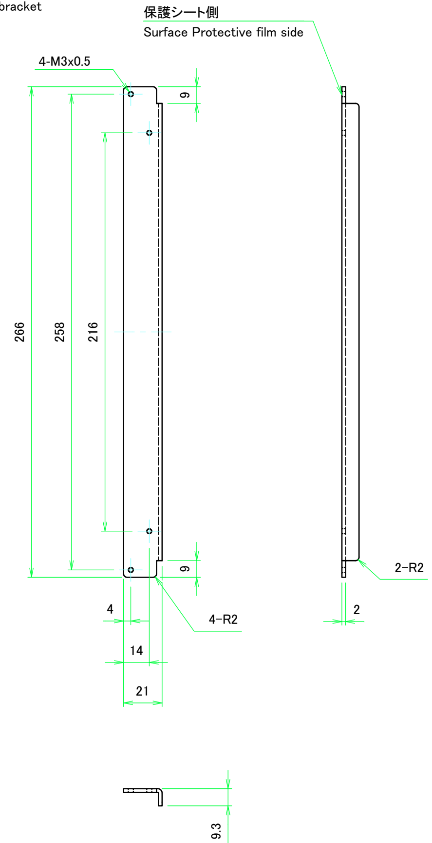
L金具 / L-bracket
