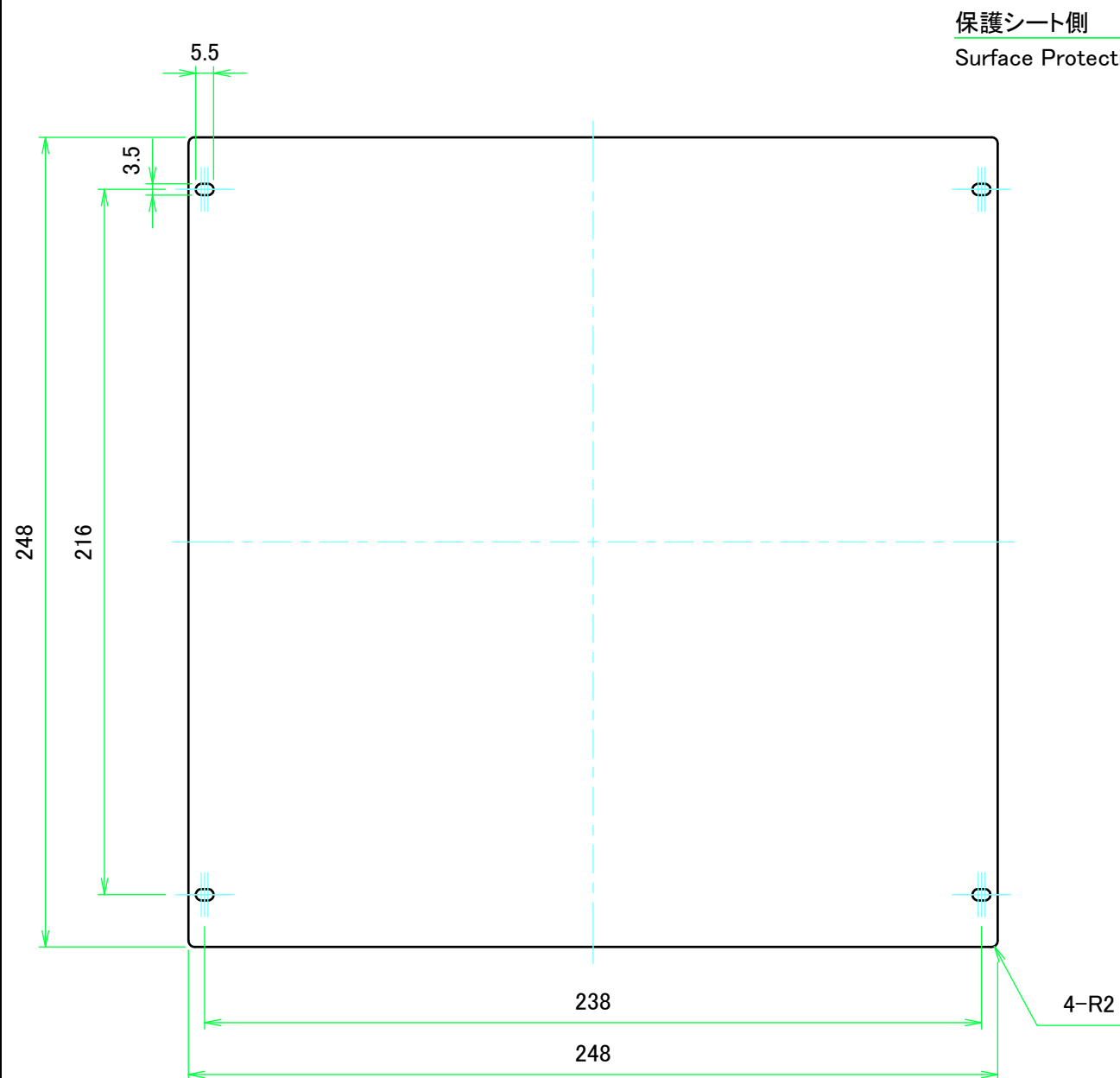
シャーシ / Mounting plate
