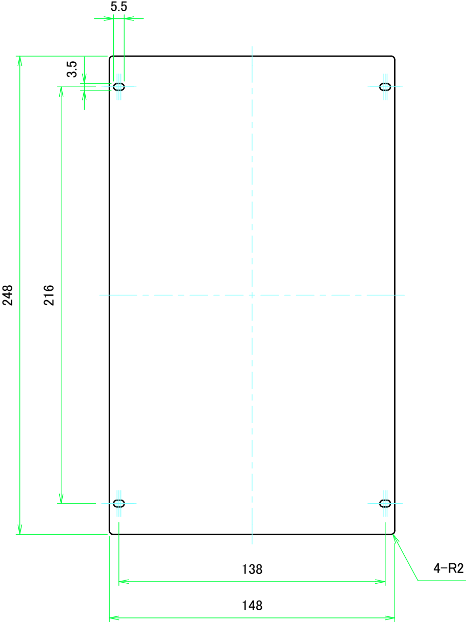
保護シート側 Surface Protective film side
