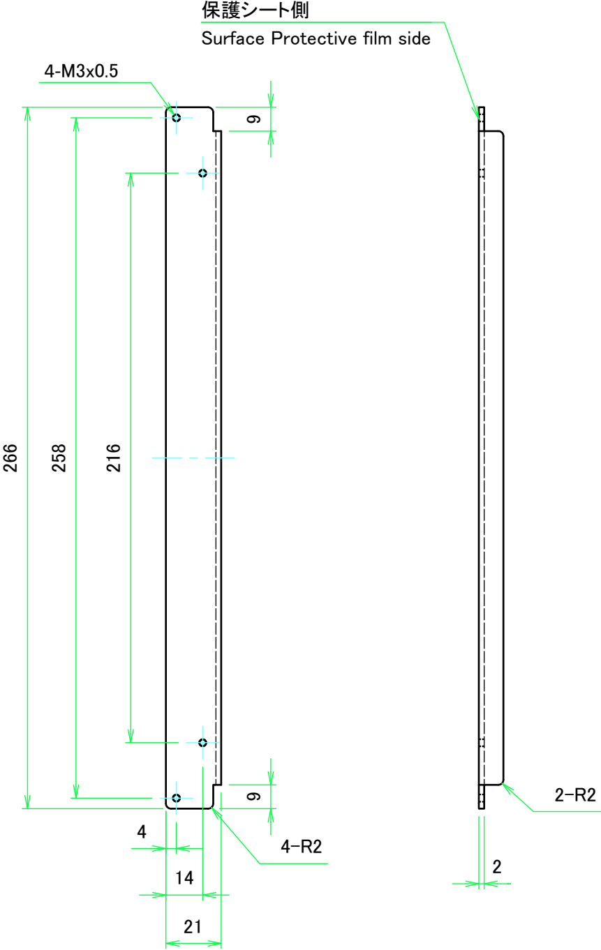
L金具 / L-bracket
