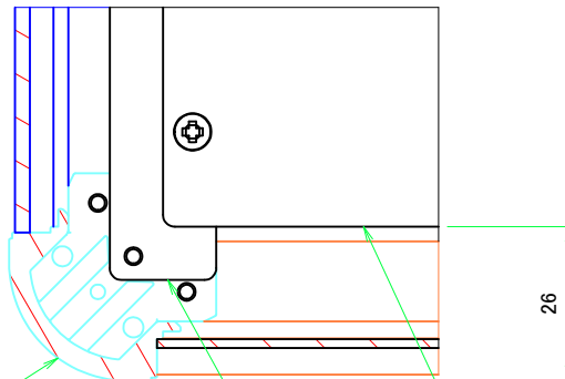
L金具 L-bracket
