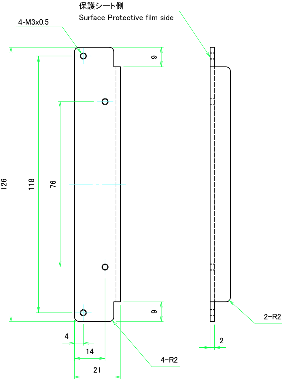
L金具 / L-bracket
