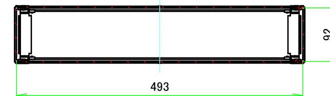
C-C ( 1 : 6.5 )
