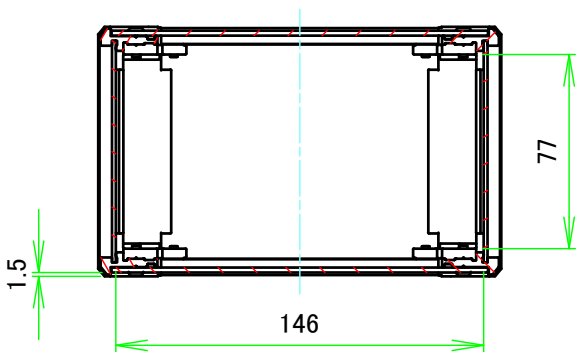
A-A ( 1 : 3 )
