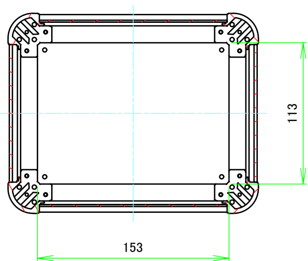
B-B ( 1 : 3 )
