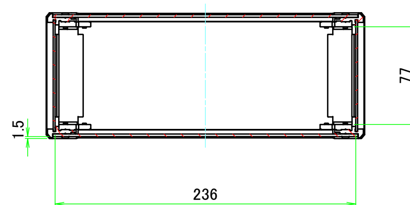
A-A (1:3)
