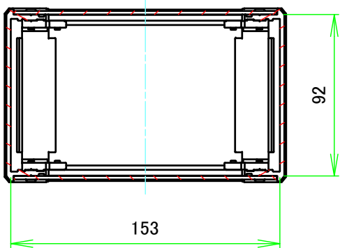
C-C ( 1 : 3 )
