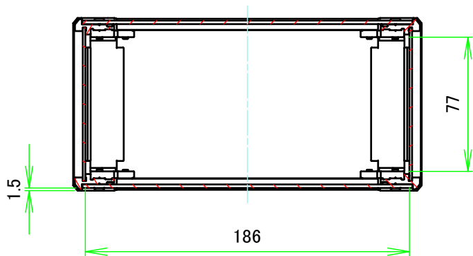
A-A ( 1 : 3 )
