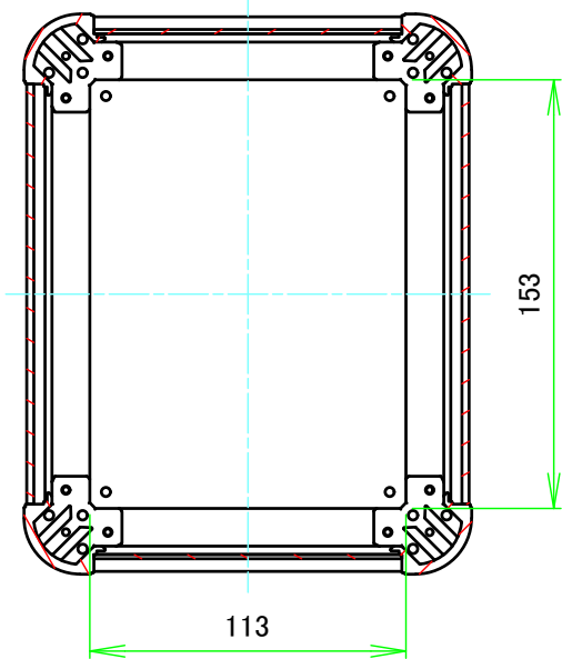
B-B ( 1 : 3 )
