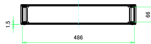
A-A (1:7)
