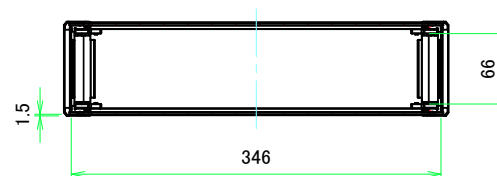
A-A (1:5)
