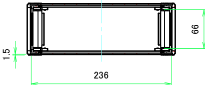
A-A ( 1 : 4.5 )
