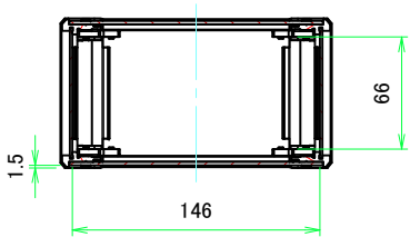
A-A (1:3.5)
