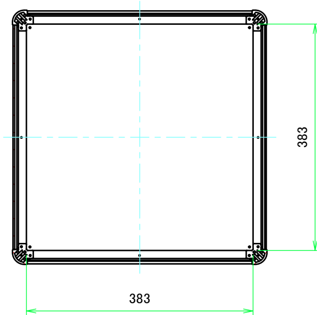
B-B ( 1:6.5 )
