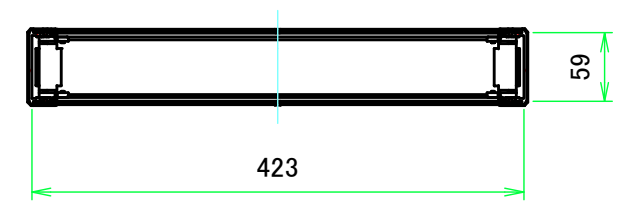
C-C ( 1:6.5 )
