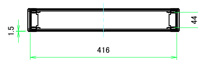
A-A ( 1:6.5 )
