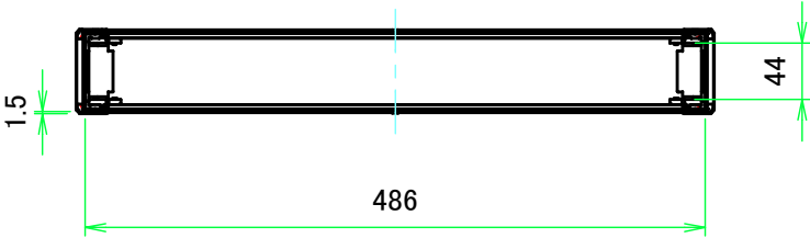
A-A ( 1:6.5 )
