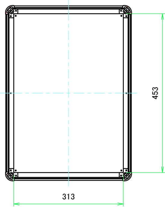
B-B ( 1:6.5 )
