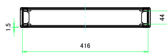
A-A (1:6)
