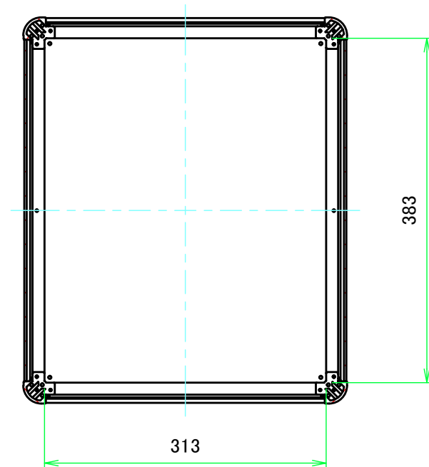
B-B ( 1:6 )
