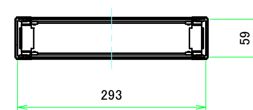
C-C ( 1:6 )
