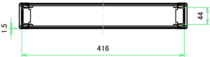
A-A ( 1:5.5 )
