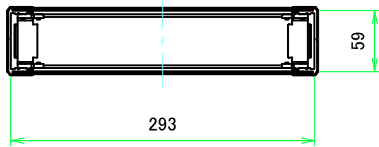
C-C ( 1:5 )
