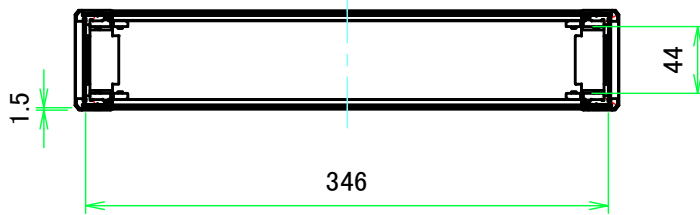
A-A ( 1:5 )
