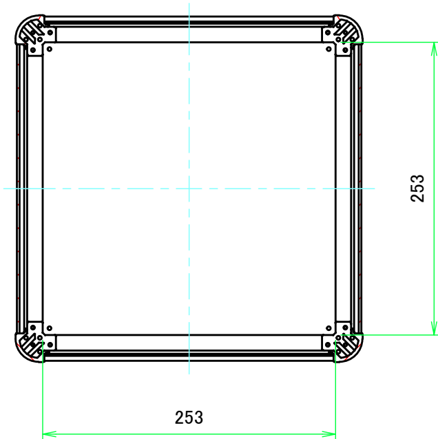
B-B ( 1:4.5 )
