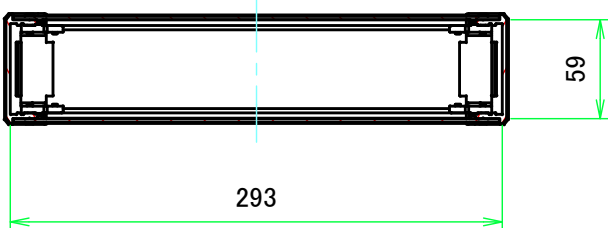
C-C ( 1:4.5 )
