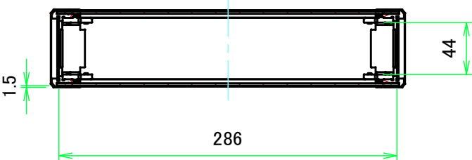
A-A ( 1:4.5 )
