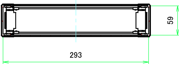
C-C ( 1:4.5 )
