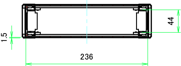
A-A ( 1:4.5 )
