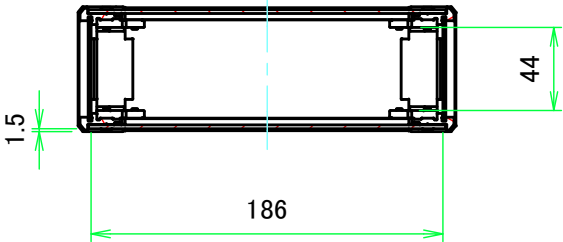
A-A ( 1:4 )
