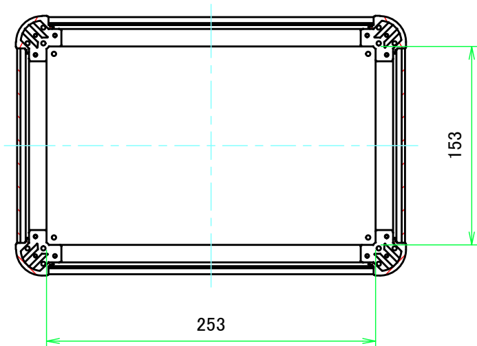
B-B ( 1:4 )
