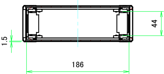
A-A ( 1:4 )
