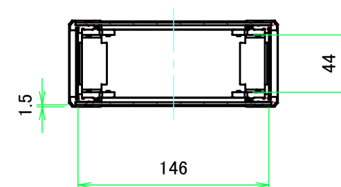
A-A ( 1:4 )
