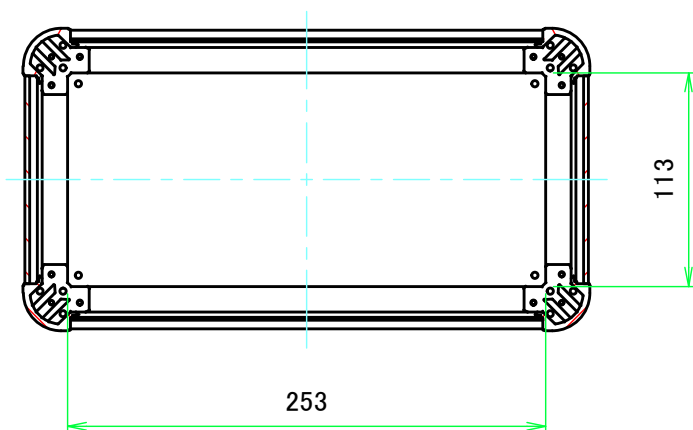
B-B ( 1:4 )
